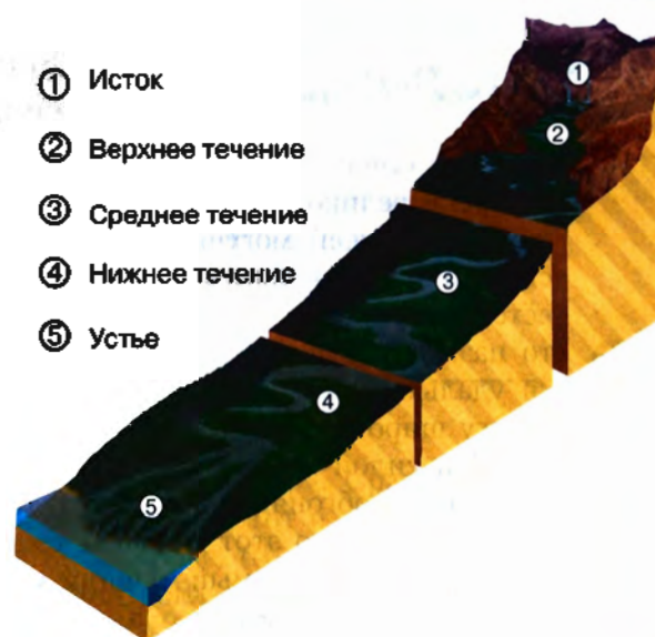
Рис. 73. Части реки
