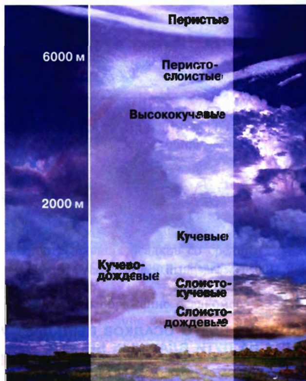
Рис. 99. Виды облаков
