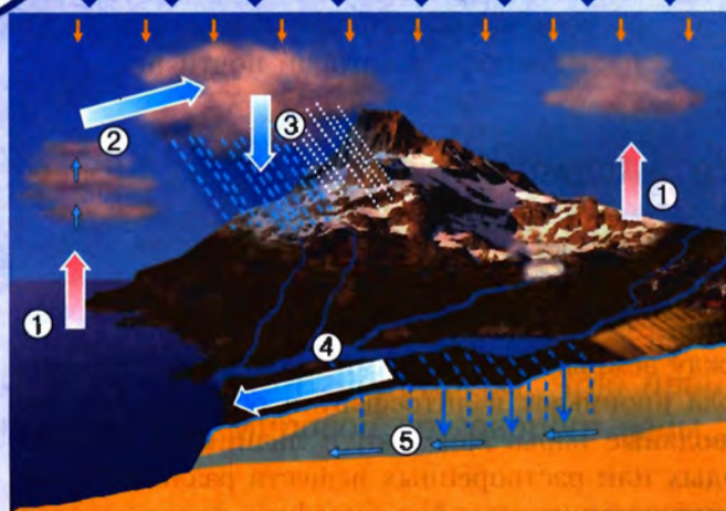
Рис. 63. Мировой круговорот воды:
