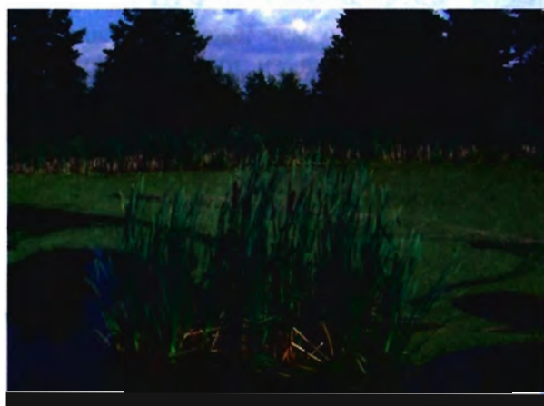
Рис. 81. Болото
