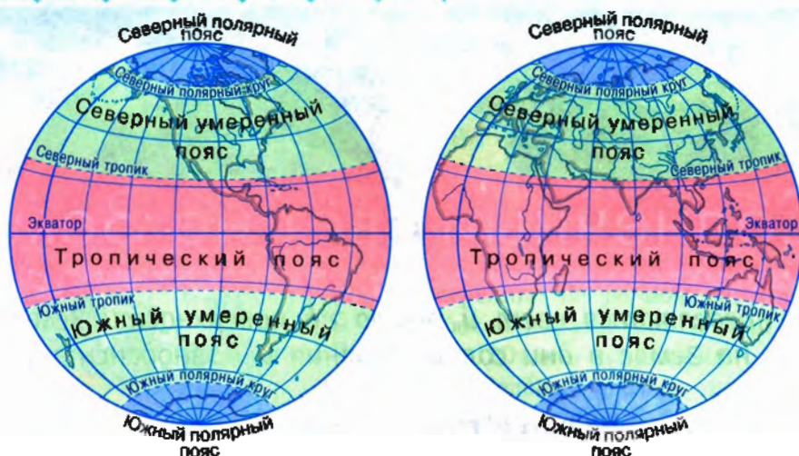
Рис. 16. Пояса освещённости
