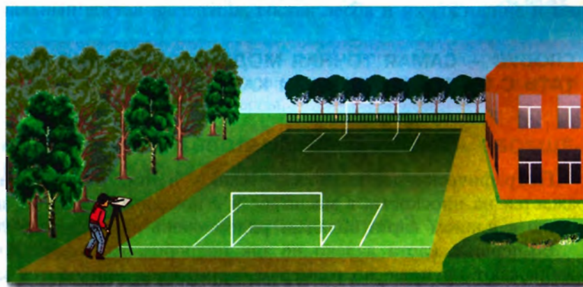
Рис. 27. Съёмка местности
