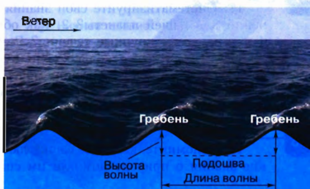
Рис. 72. Схема волны
