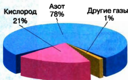
Рис. 86. Состав воздуха
